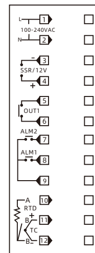
外形尺寸及接线示例 External Dimensions and Wiring Example
